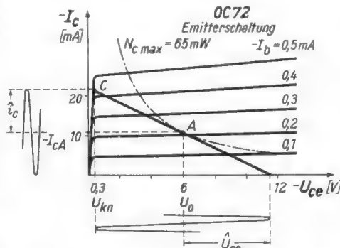
Bild 2. I_c/U_{ce} -Kennlinienfeld des Transistors OC 72 in Emitterschaltung
