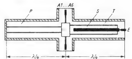
Bild 4. Prinzip des Sechsfach-Verteilers
