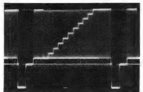
Bild 5. Oszillogramm des elektronischen Testbildes über die Zeile
