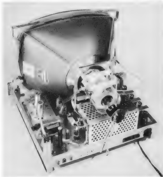
Bild 4. Chassis des T 604 mit Bildröhre MW 43-69
