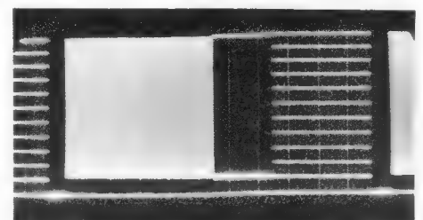
Bild 6. Oszillogramm des elektronischen Testbildes über das Bild
