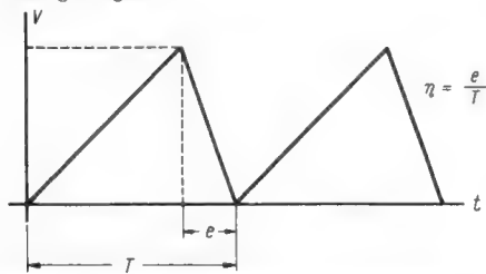
Bild 2. Kurvenform der Sägezahnspannung für das im Text erwähnte Beispiel
