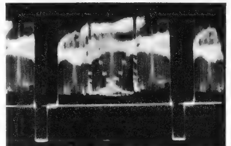
Bild 3. Oszillogramm des Universal-Testbildes über die Zeile
