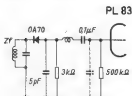
Bild 1. Prinzip einer Video-Demodulatorstufe
