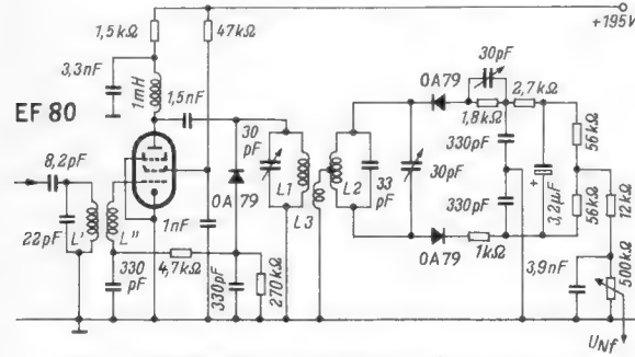
Bild 5. Ratiodetektor mit geregelter Zf-Stufe für die Vorunterdrückung
