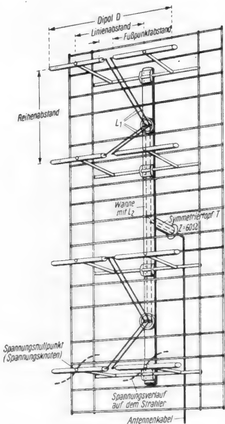
Bild 1. Antennenfeld mit vier Ganzwellendipolen
