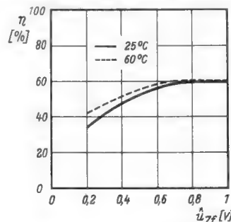
Bild 2. Gleichrichtereffekt \eta bei kleinen Signalspannungen und verschiedenen Temperaturen (OA 70, R = 3,9 k \Omega )
