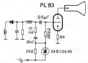
Bild 8. Praktisch ausgeführte Schwarzpegelstufe
