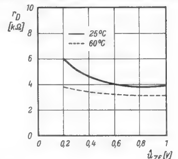
Bild 3. Dämpfungswiderstand r_D bei kleinen Signalspannungen und verschiedenen Temperaturen (OA 70, R = 3,9 k \Omega )
