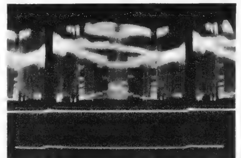
Bild 4. Oszillogramm des Universal-Testbildes über das Bild
